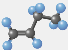
1-Butene copolymere
