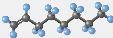
1-Octene copolymere
