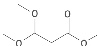
Methyl 3,3-dimethoxypropionate Cas No: 7424-91-1
